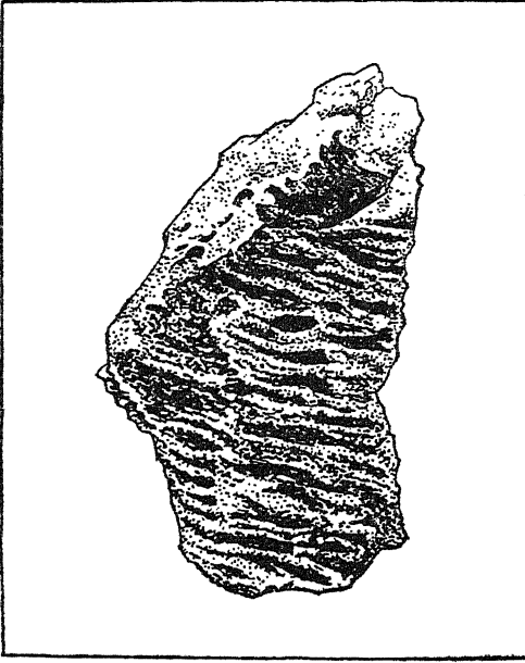
चित्र १९९—वायुक्षरित मलानी रायोलाइट, जोधपुर के पास
